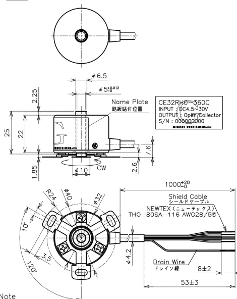
Fig.1 Dimension 寸法
