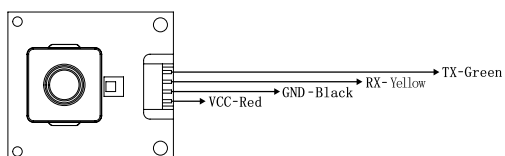
UART TTL 3.3V
