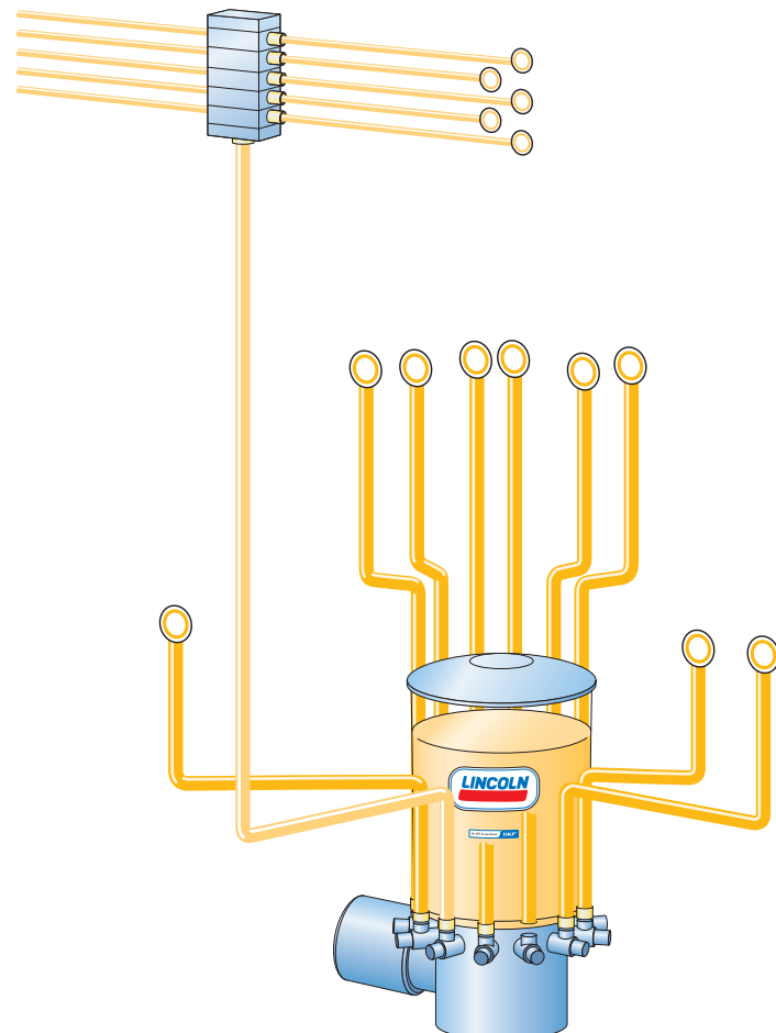
Schemazeichnung Mehrleitungsanlagen
