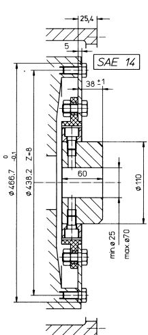
CF-K-150 SAE 14
