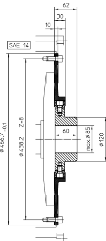
CF-K-200 SAE 14
