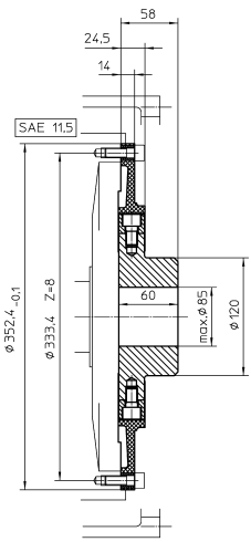
CF-K-200 SAE 11,5
