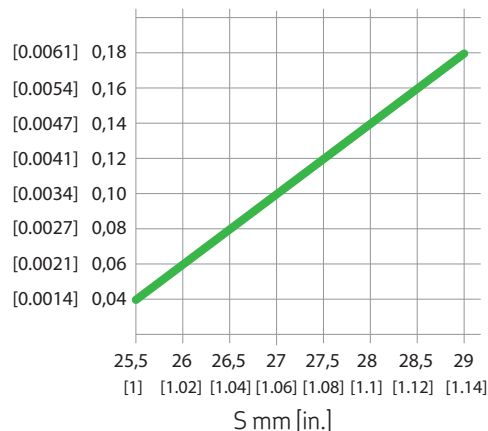
Einstellen der Fördermenge am Pumpenelement R Abb. 11
