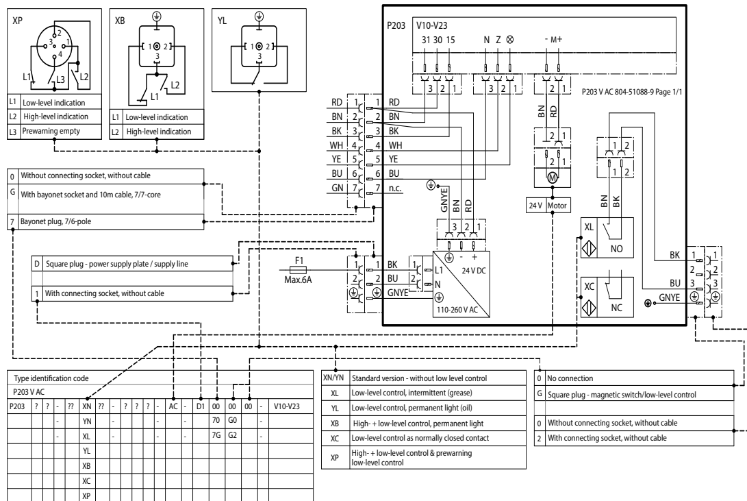
Anschlussplan P203 V AC mit Steuerplatine V Abb. 44
