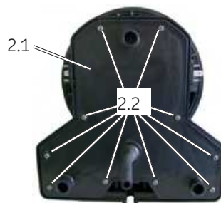
Gehäusedeckel abschrauben Abb. 21
