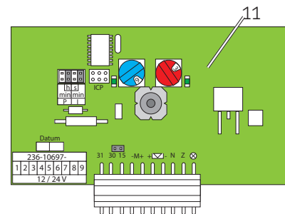
Steuerplatine entnommen Abb. 23
