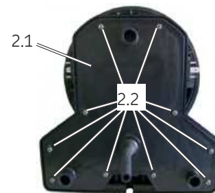
Gehäusedeckel montieren Abb. 26
