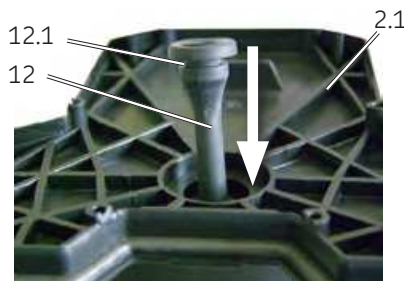
Entwässerungsschlauch montieren Abb. 24
