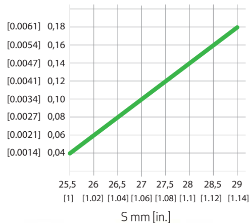
Einstellen der Fördermenge am Pumpenelement R Abb. 10
