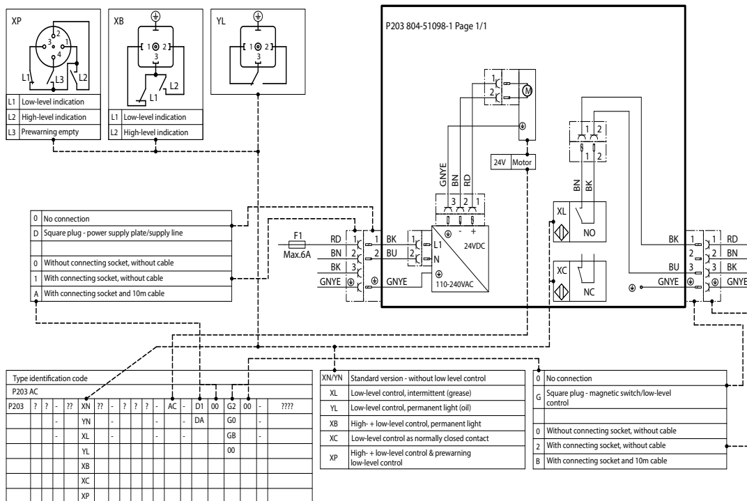
Anschlussplan P203 V AC ohne Steuerplatine Abb. 32
