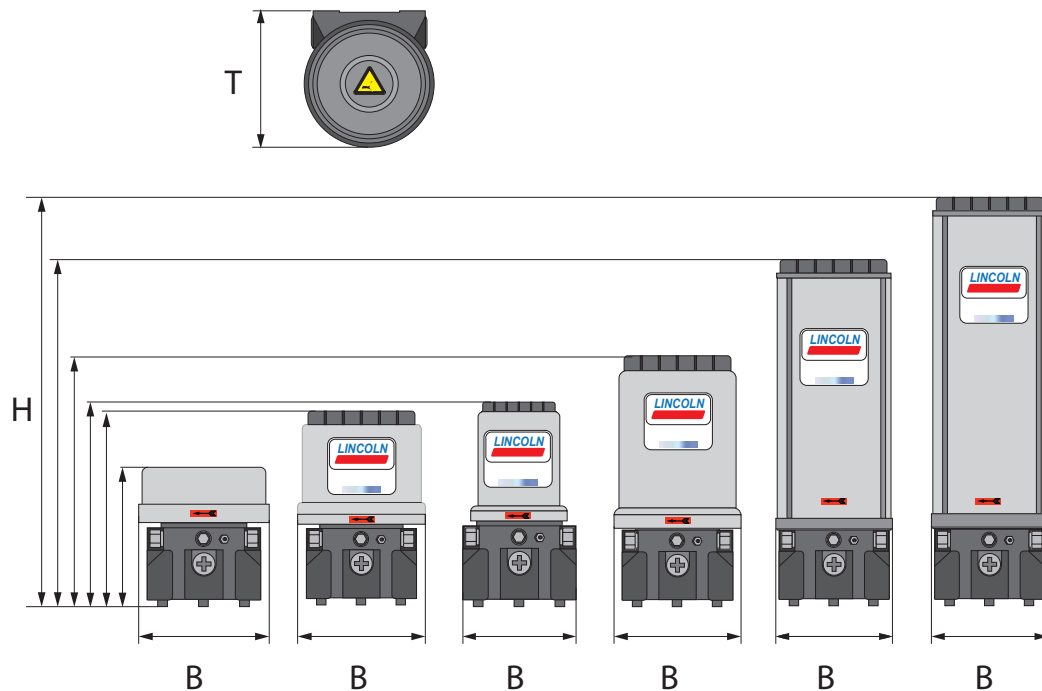
Mindesteinbaumaße Abb. 5
