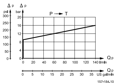
Kennlinie des Umlaufdrucks in Neutralstellung (Open Center)
