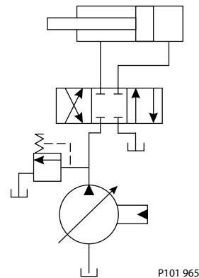
Einfacher Closed-Center-Kreislauf
