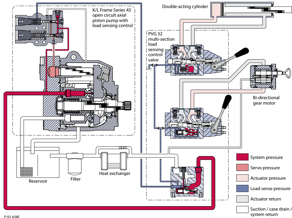
Schaltbild
