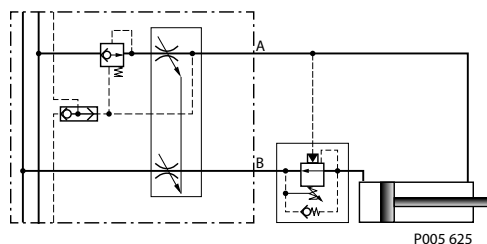
Abb. 4 Durchflussgeregelter Schieber
