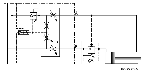
Abb. 5 Druckgeregelter Schieber
