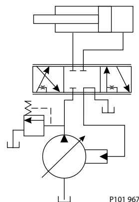
Load-Sensing-System
