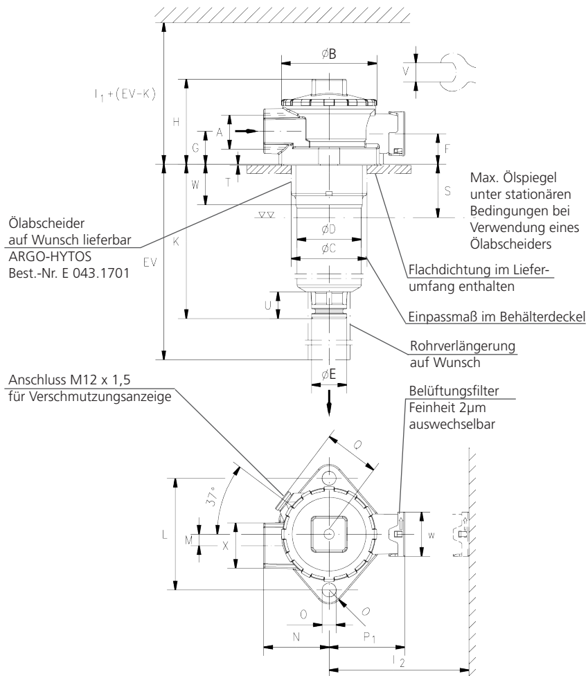
Ausführung mit Belüftungsfilter
