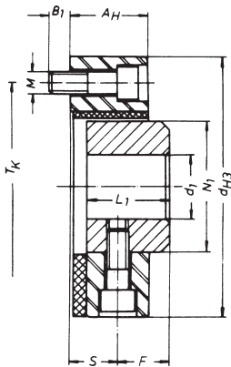
Bauform / type 1
