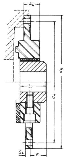
Bauform / type 4
