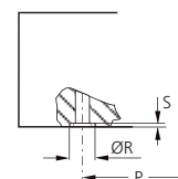
Bohrungen p_1 / p_2 p_1 = höherer stat. Druck p_2 = niedriger stat. Druck
