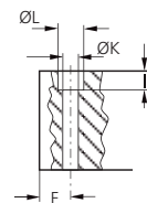
Befestigungsbohrungen
