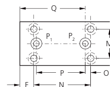
Flanschbild
