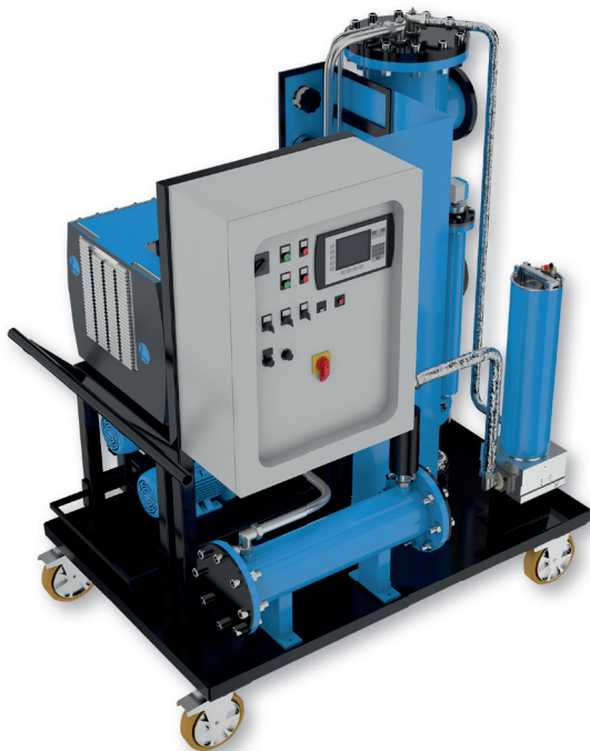
Entwässerungssystem OPS 550
