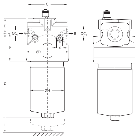
Gewindeanschluss
