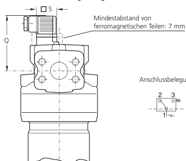
Ausführung mit integrierter elektr. Verschmutzungsanzeige
