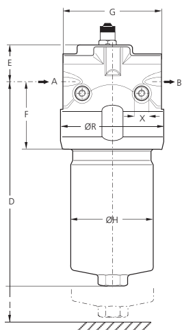
Flanschanschluss
