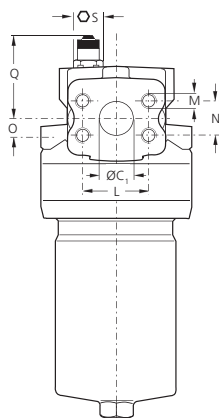
Ausführung mit integrierter elektr. Verschmutzungsanzeige
